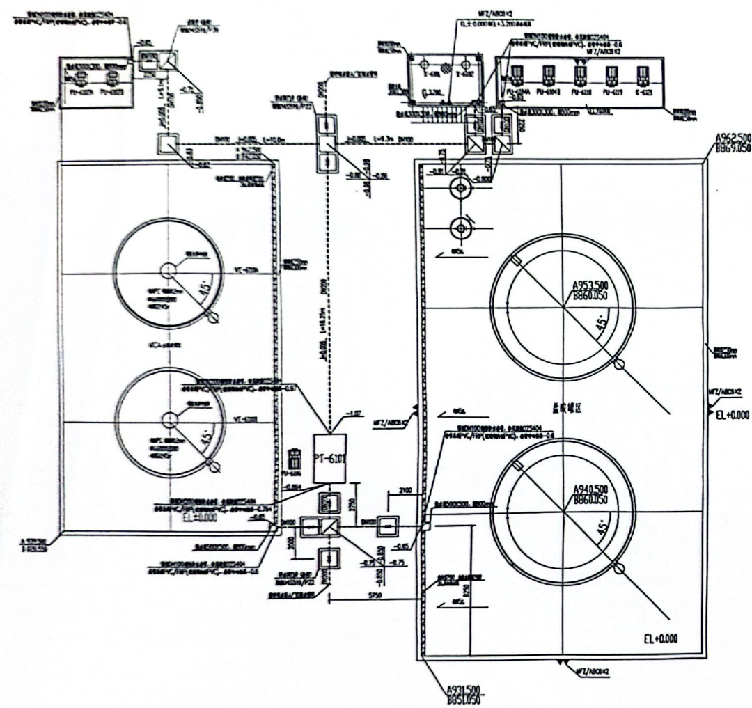
室外消火及消防平面布置图 1:100
